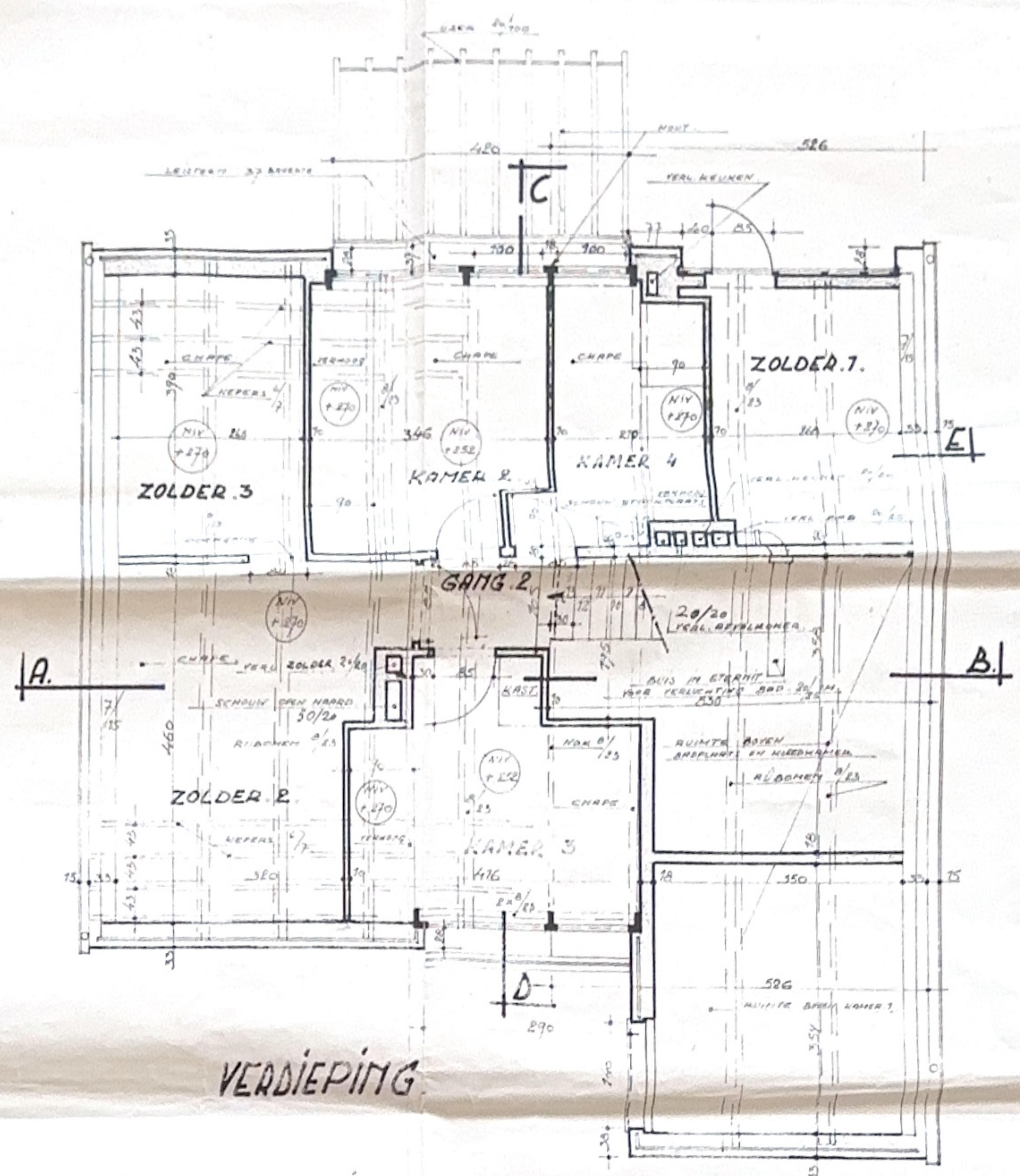
LIGGINGSPLAN
