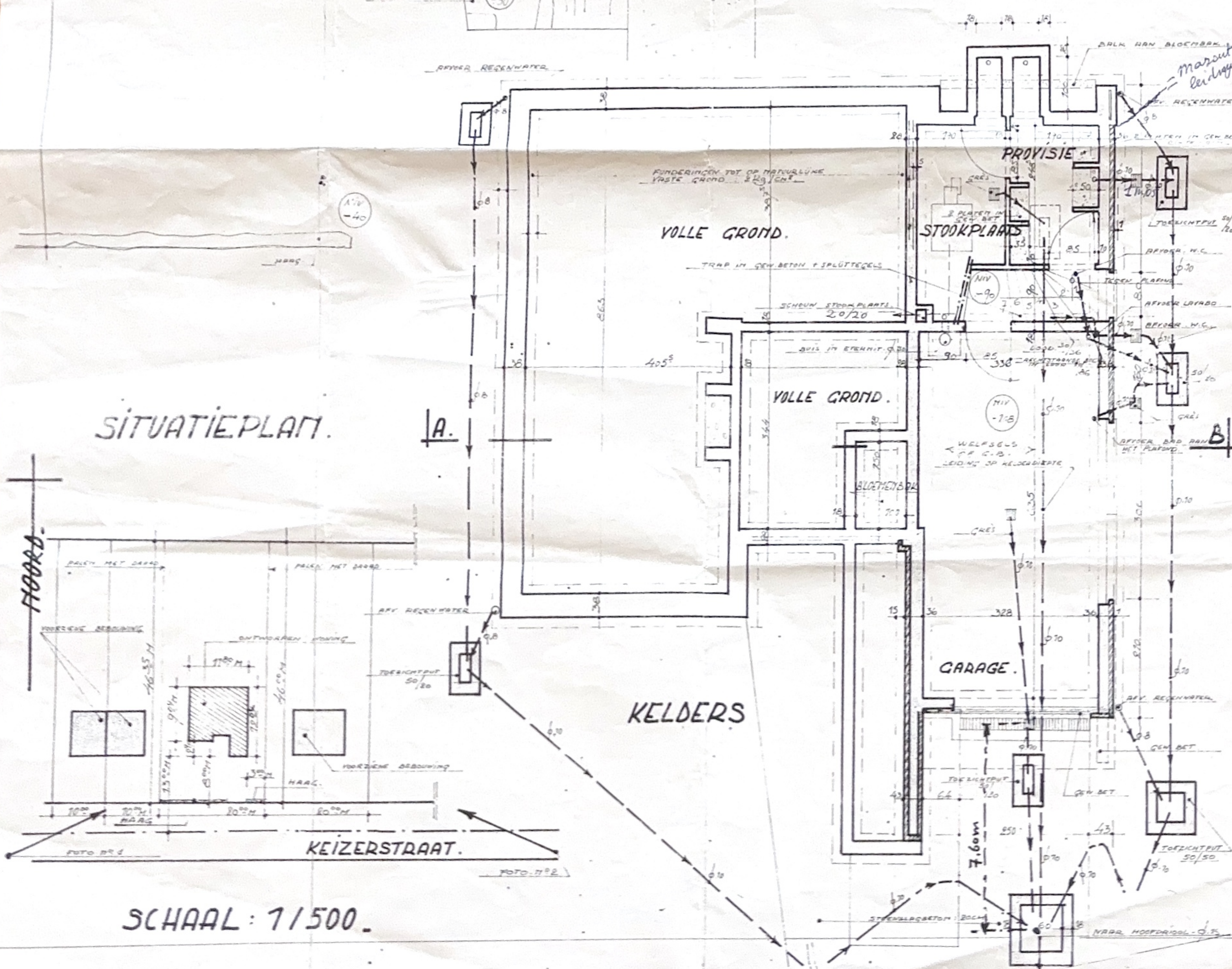
GRONDPLANS.
